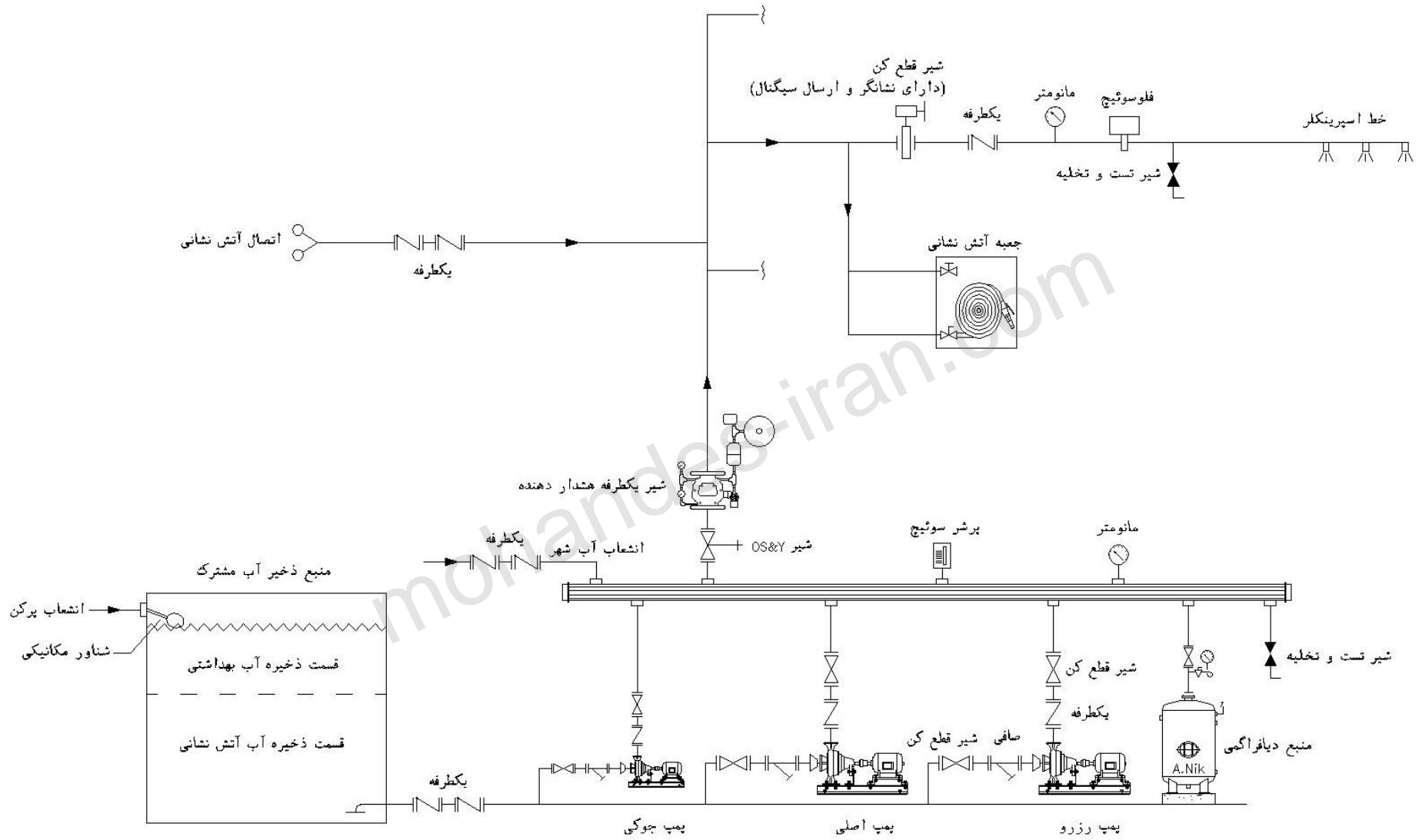
شکل ۱-۵۹- نمای شماتیک یک سیستم اطفای حریق نمونه
